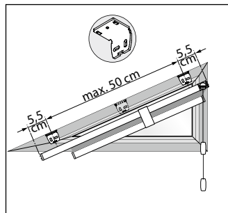
WANDWINKEL FÜR FD SLOPE 3 WALL FIXING BRACKET FOR FD SLOPE 3 – SUPPORT MURAL POUR FD SLOPE 3
